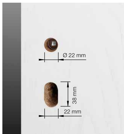
preparazione della porta per guarniture con mini-rosette HOPPE con bocchetta
