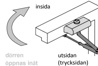
Fig. 61: trycksida karmmontage
