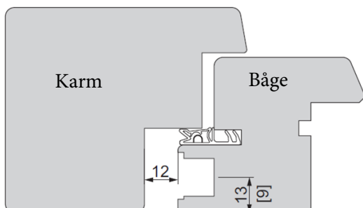
Överfals & beslagsdjup
