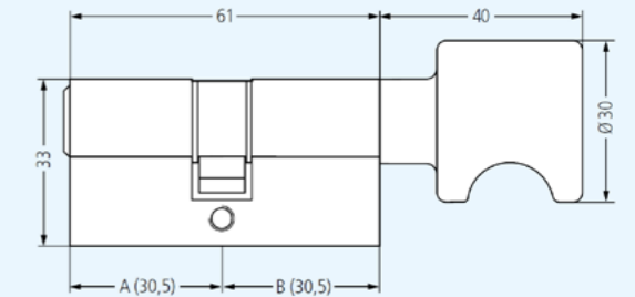
Winkhaus profil/euro cylinder med knapp/vred Key One XPERT.
